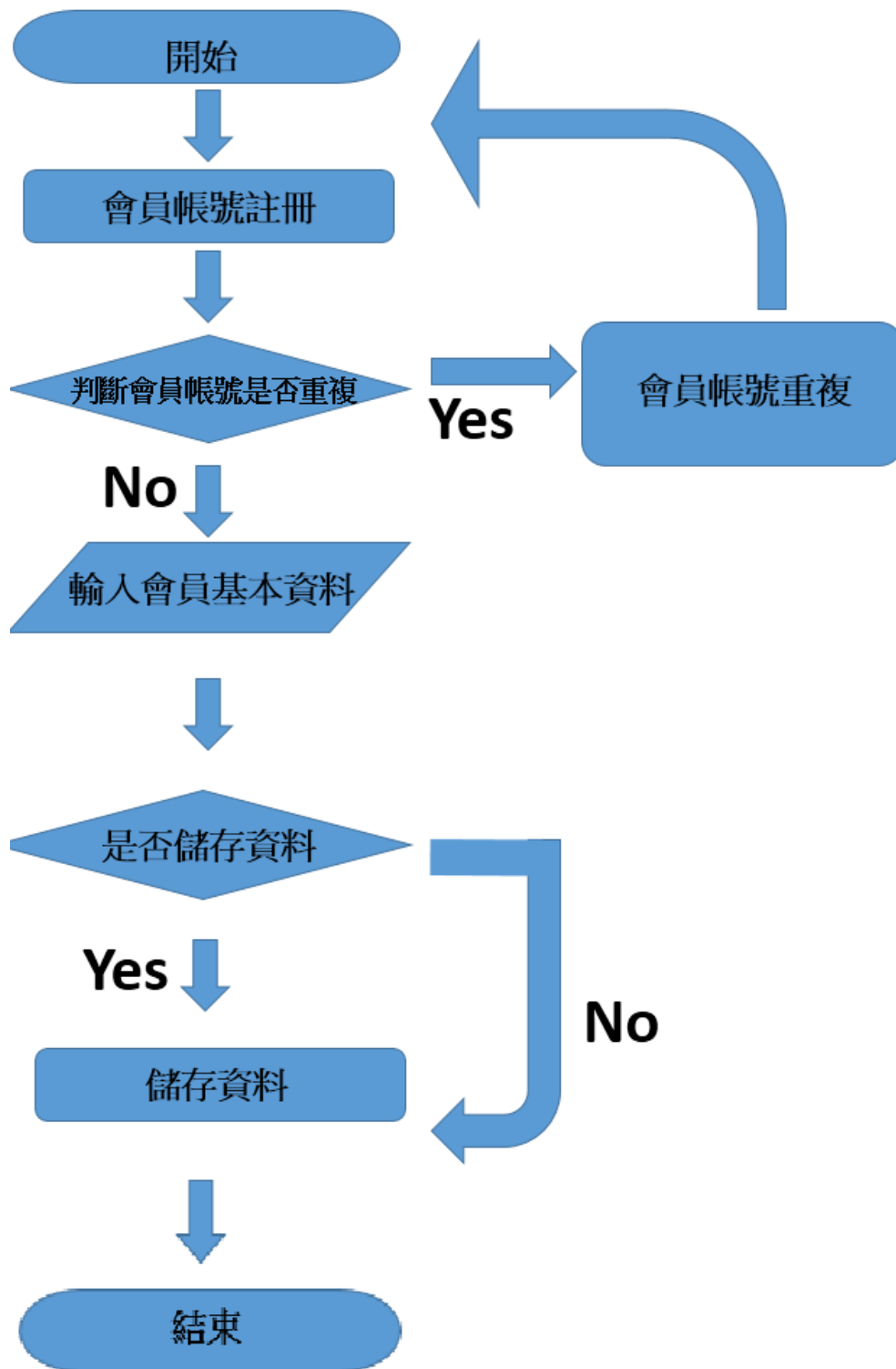
圖 3.3 註冊會員流程圖
