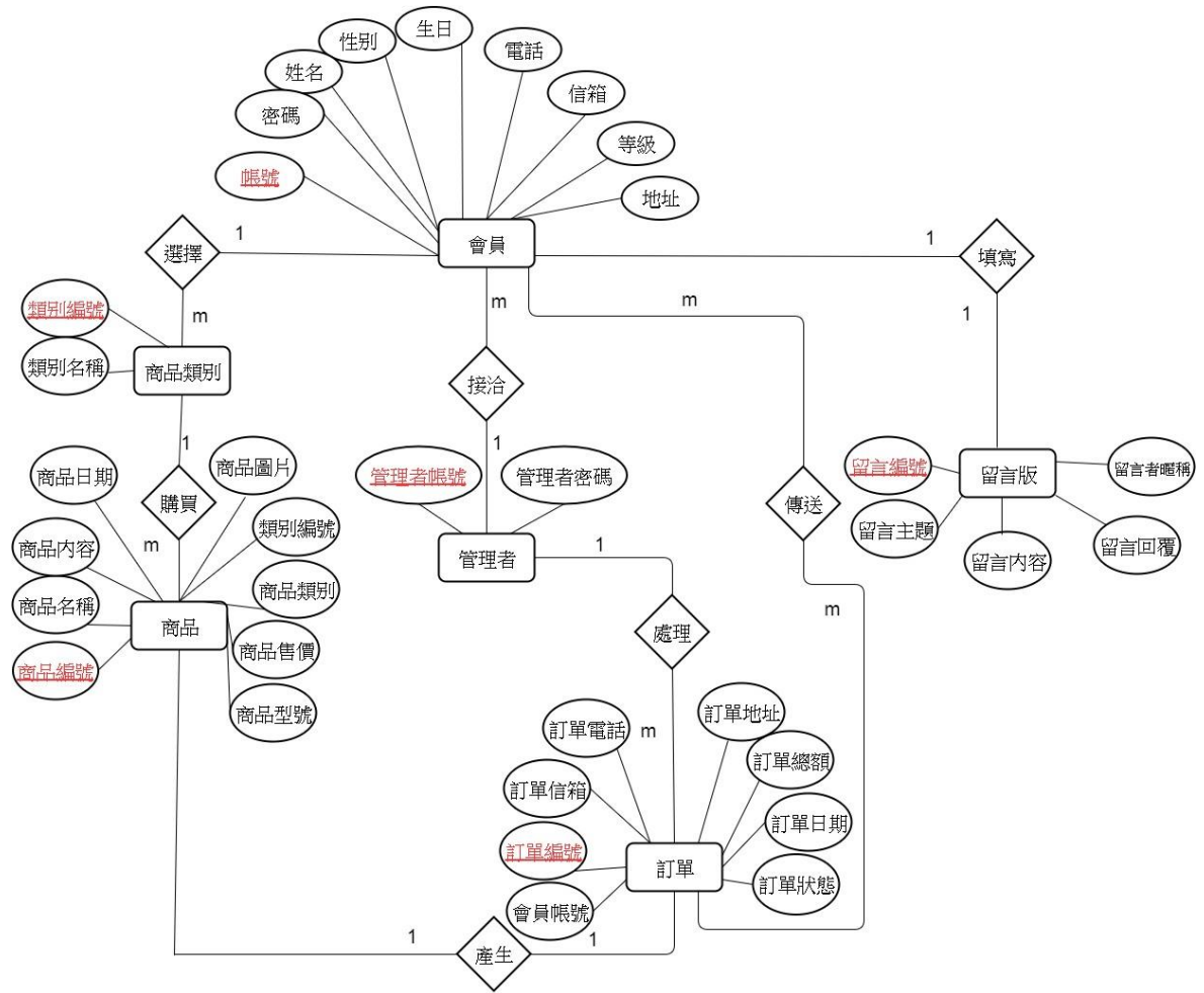
圖 3.7 E-R model 圖
