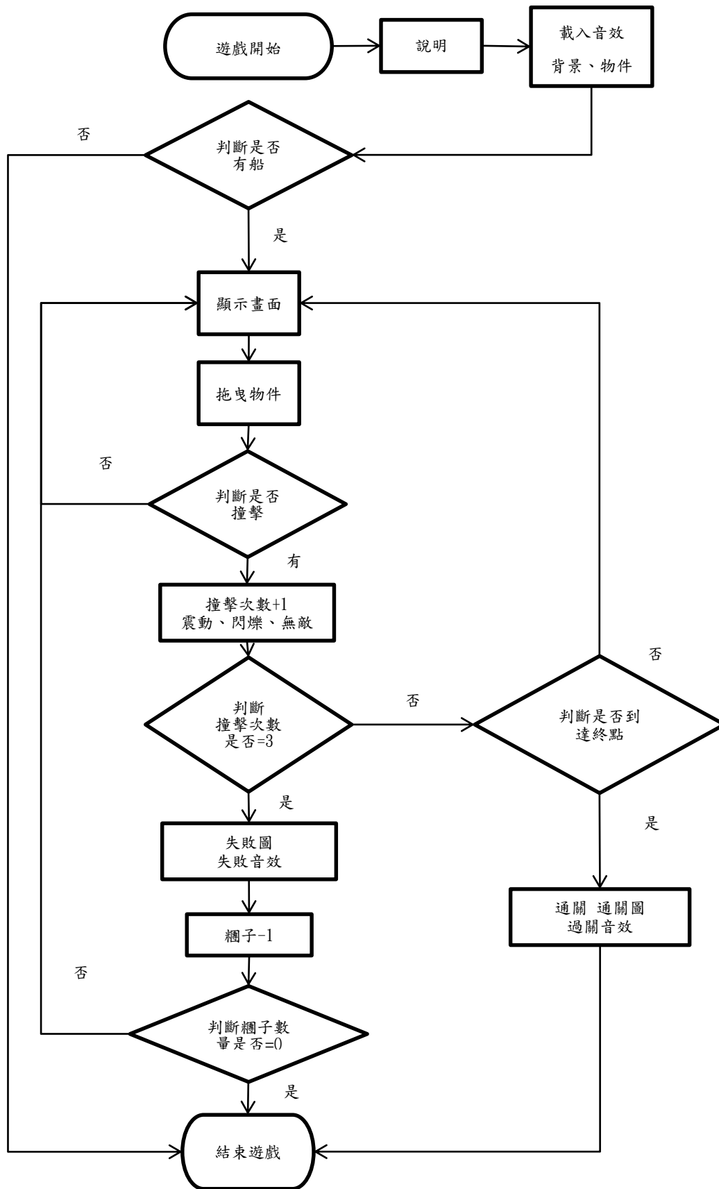
圖 3-2-9-6：勇闖惡魔島流程圖
