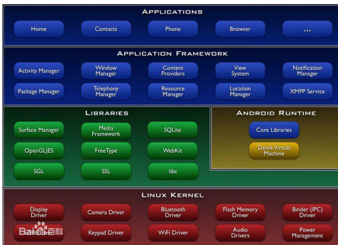
圖 2-3-1：Android 系統架構參考圖【3】
