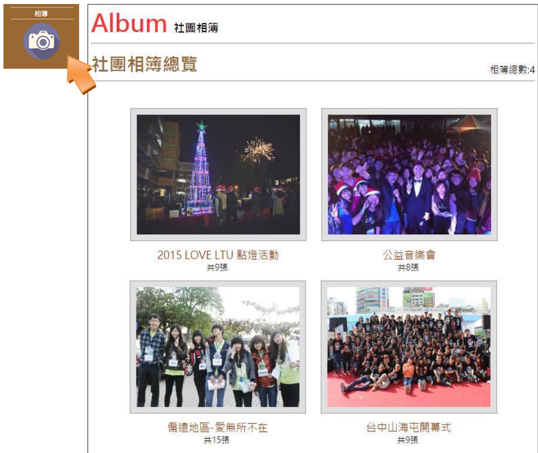
圖 4-20 相簿
