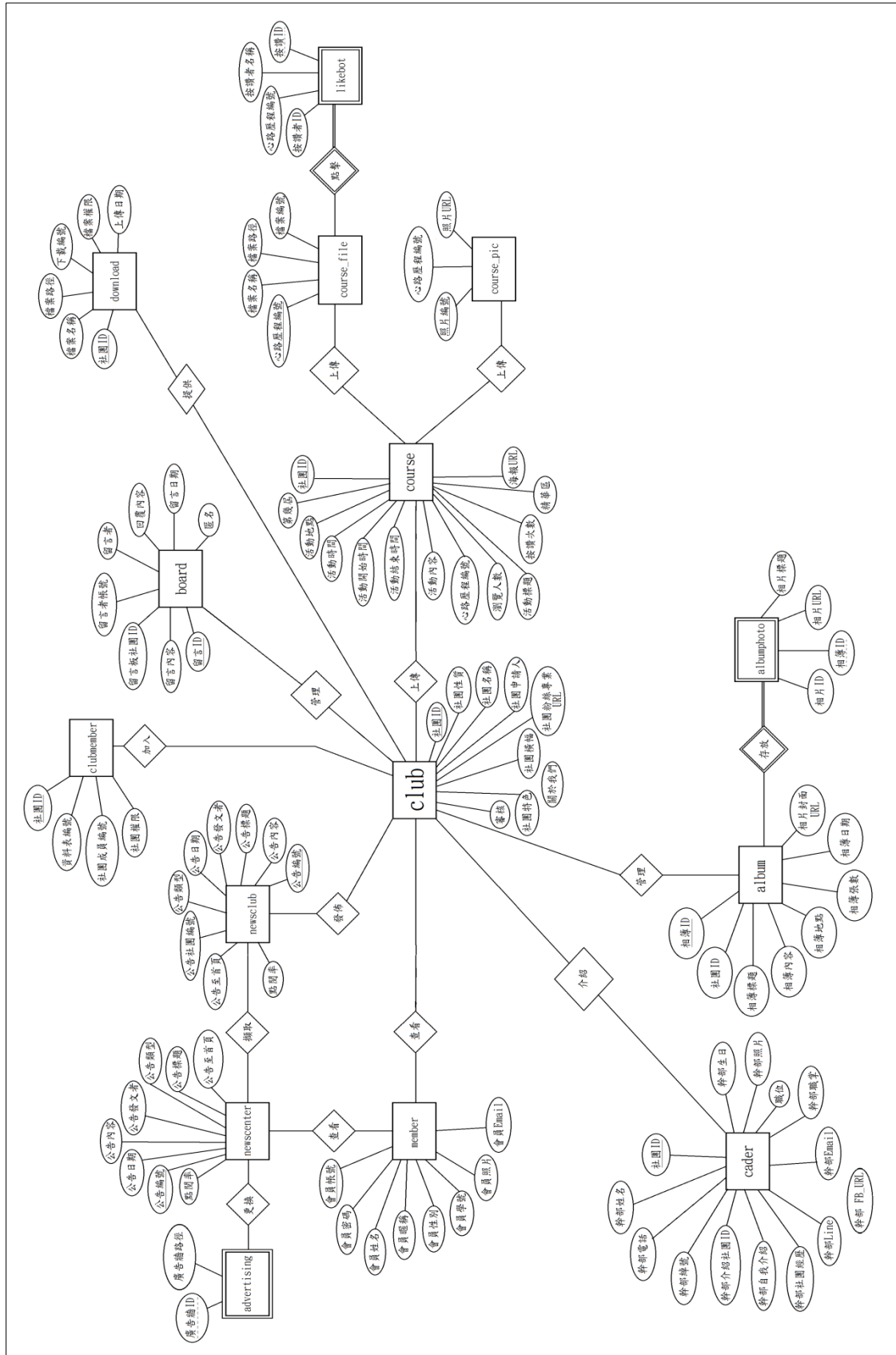
圖 3-7 專題 ER-Model 圖
