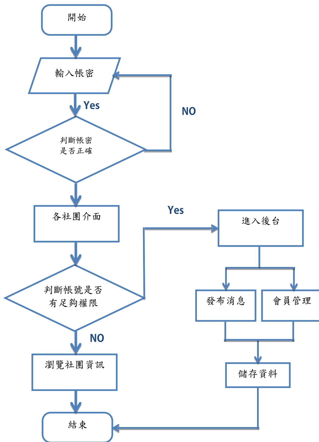
圖 3-3 登入流程圖
