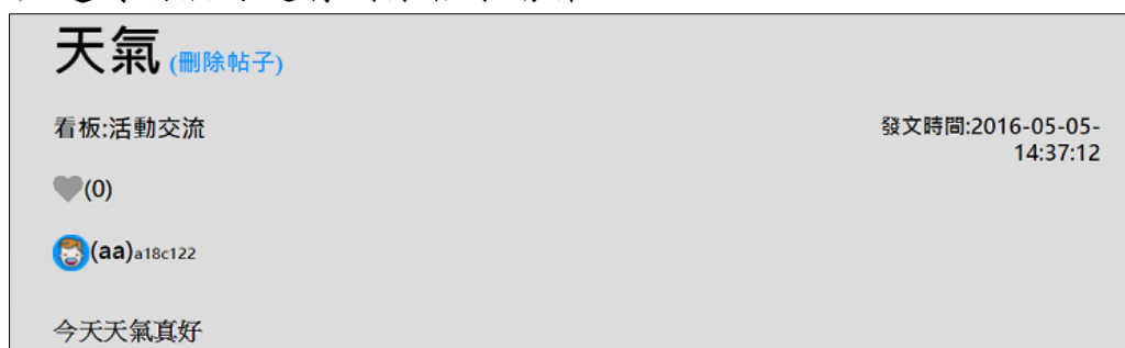
圖 4-58 刪除帖子
