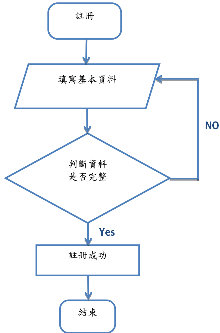
圖3-5 註冊流程圖
