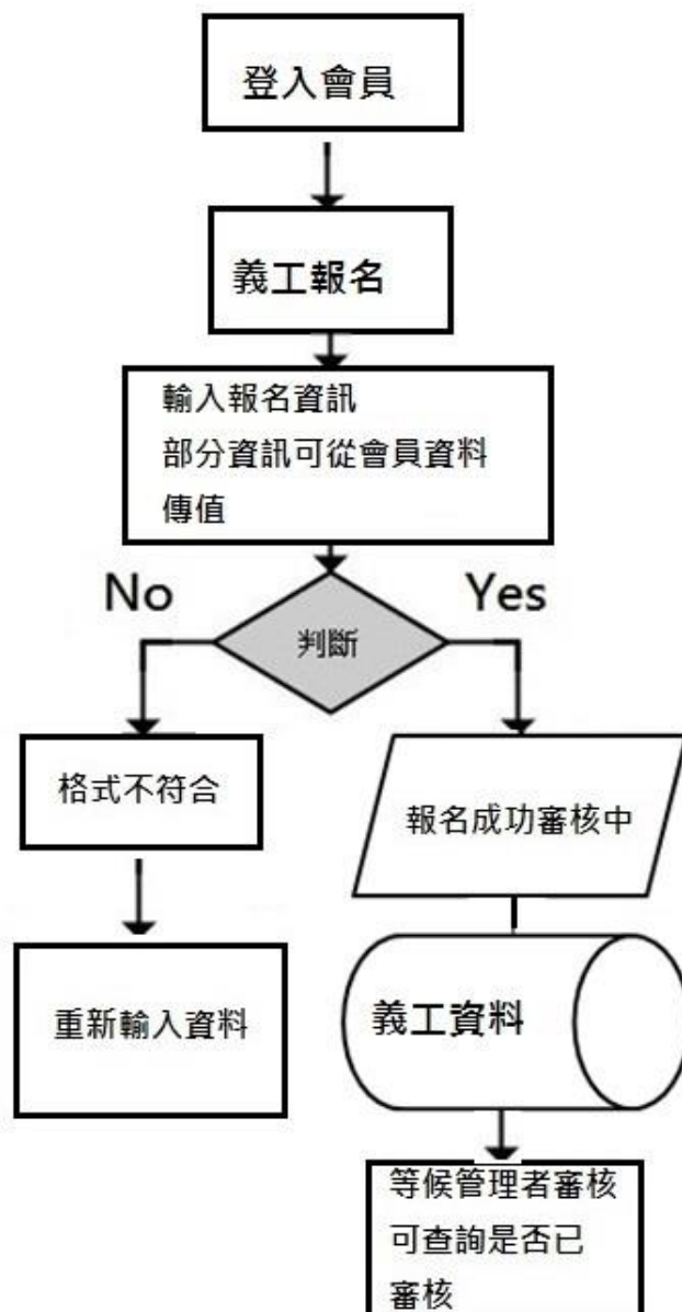
圖 3.5 義工報名流程圖
