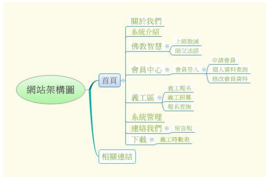
圖 3.2 網站架構圖
