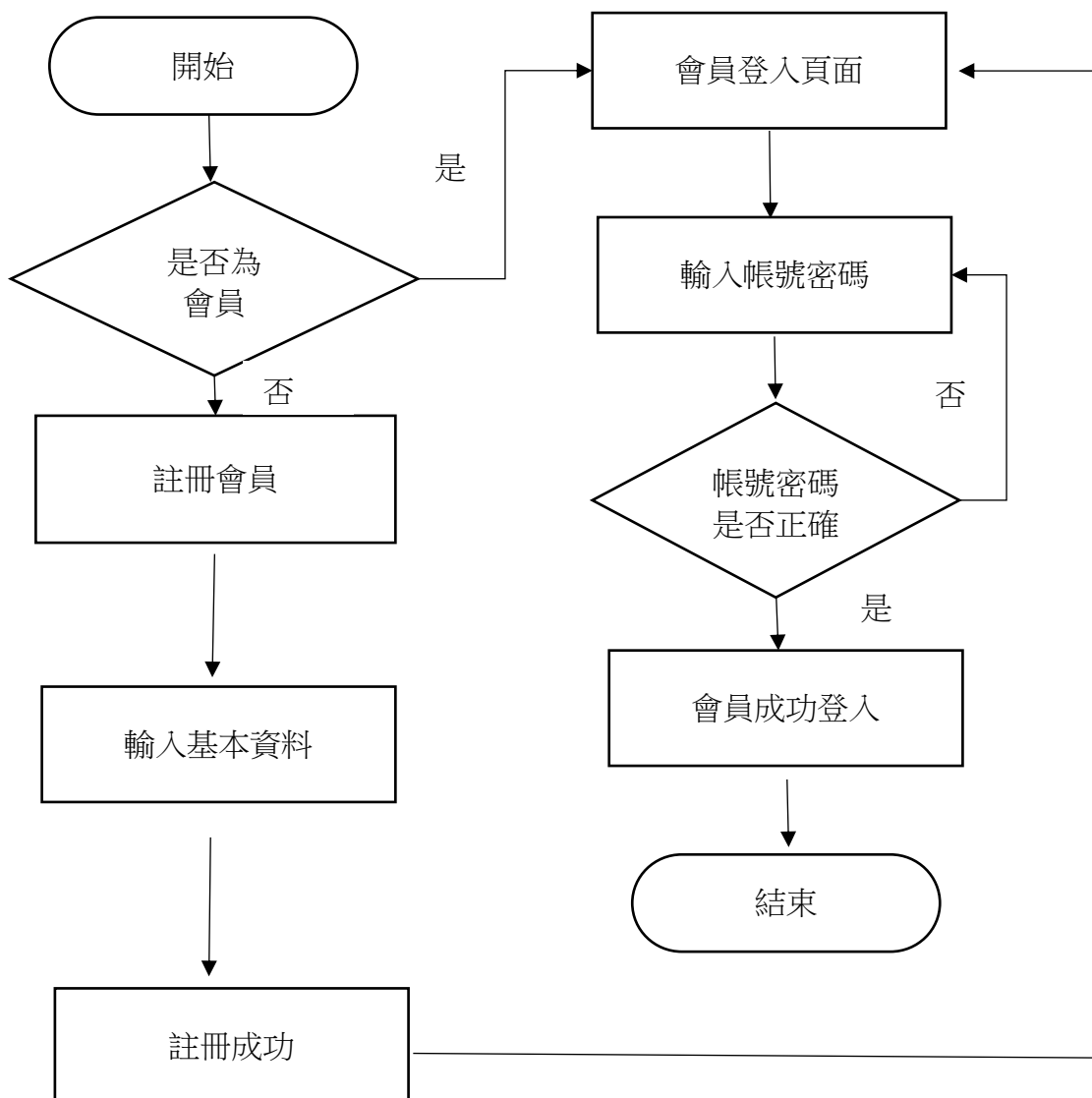
圖 3.3 註冊、登入流程圖
